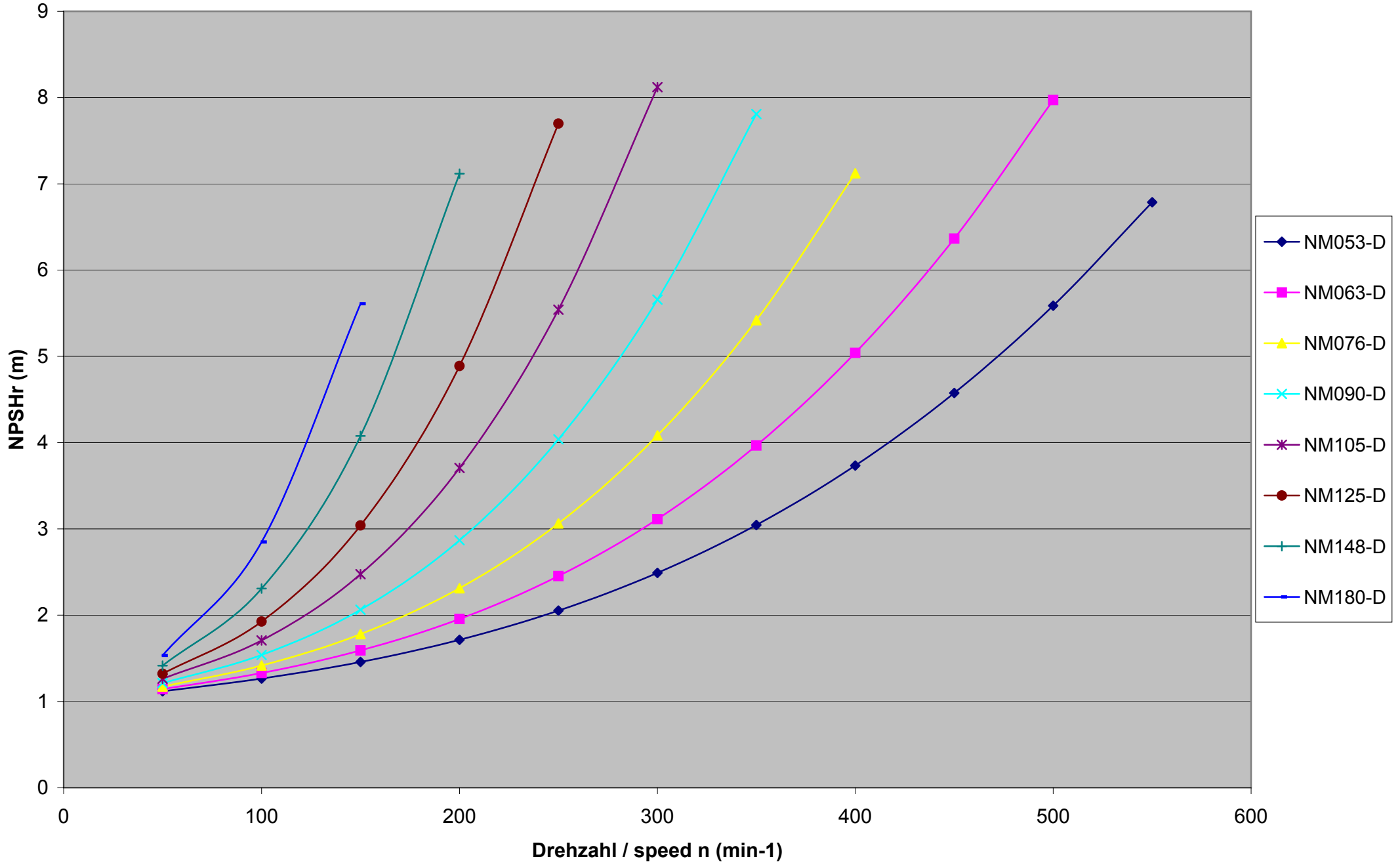
NPSHr-Werte abh. von Drehzahl n für NM-Reihe, D-Geom. / NPSHr values vs. speed n for NM series, D geom.
